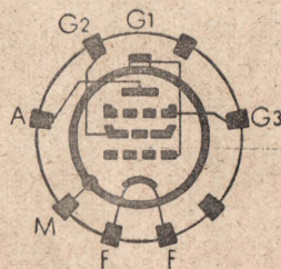
Sockelschaltung
